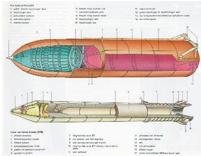
Uzay Mekiđi sıvı ve katı yakıt tankları
