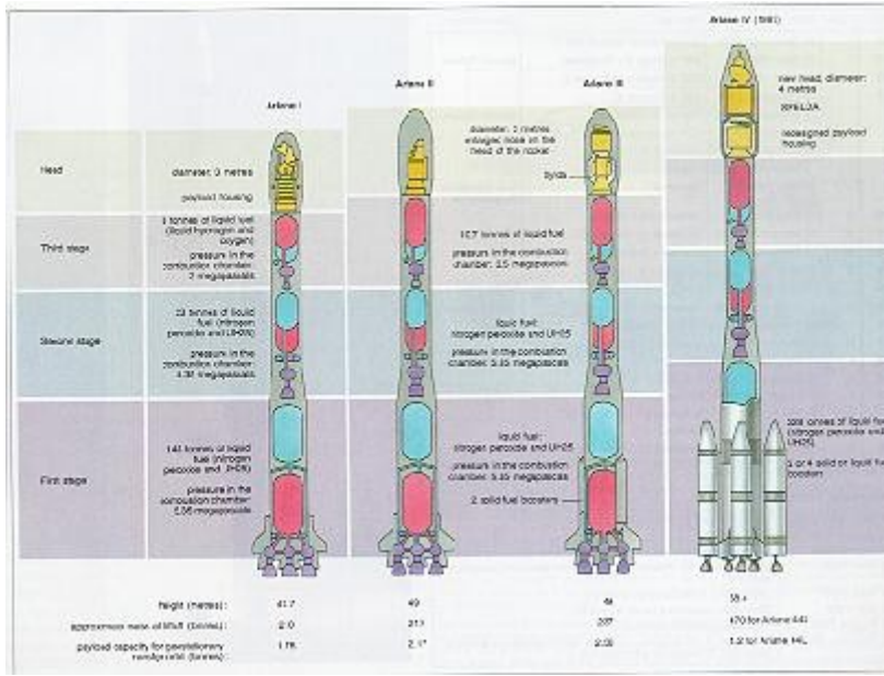
Ariane Uydü Fırlatma Araçları
